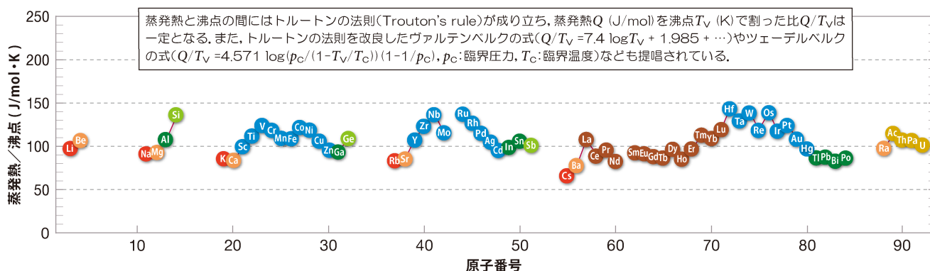
図1 各元素の蒸発熱。
