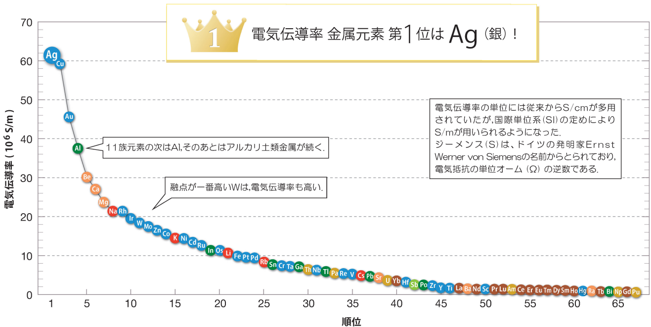
図2 金属元素の電気伝導率ランキング(67位まで).
