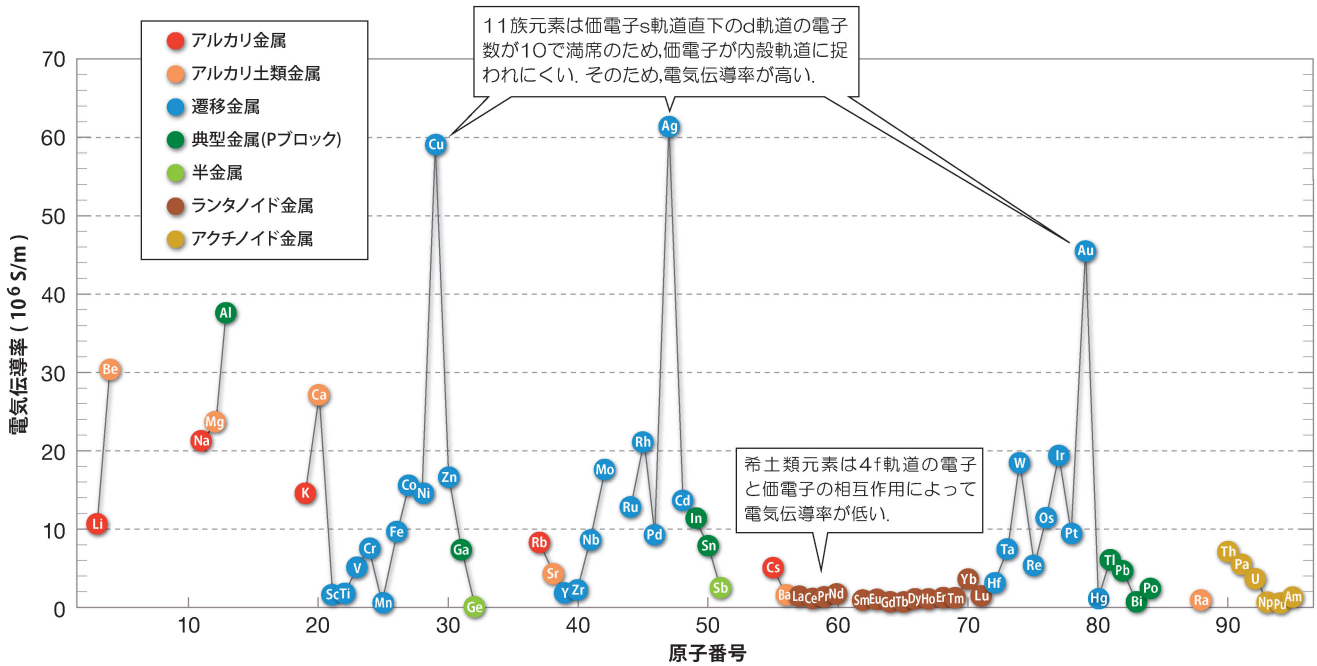
図1 各元素の電気伝導率.
