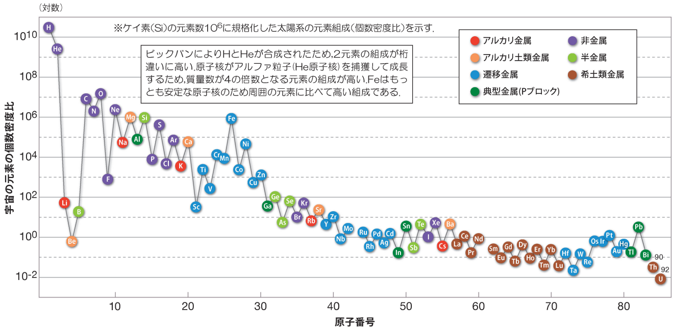
図1 各元素の宇宙の元素組成.
