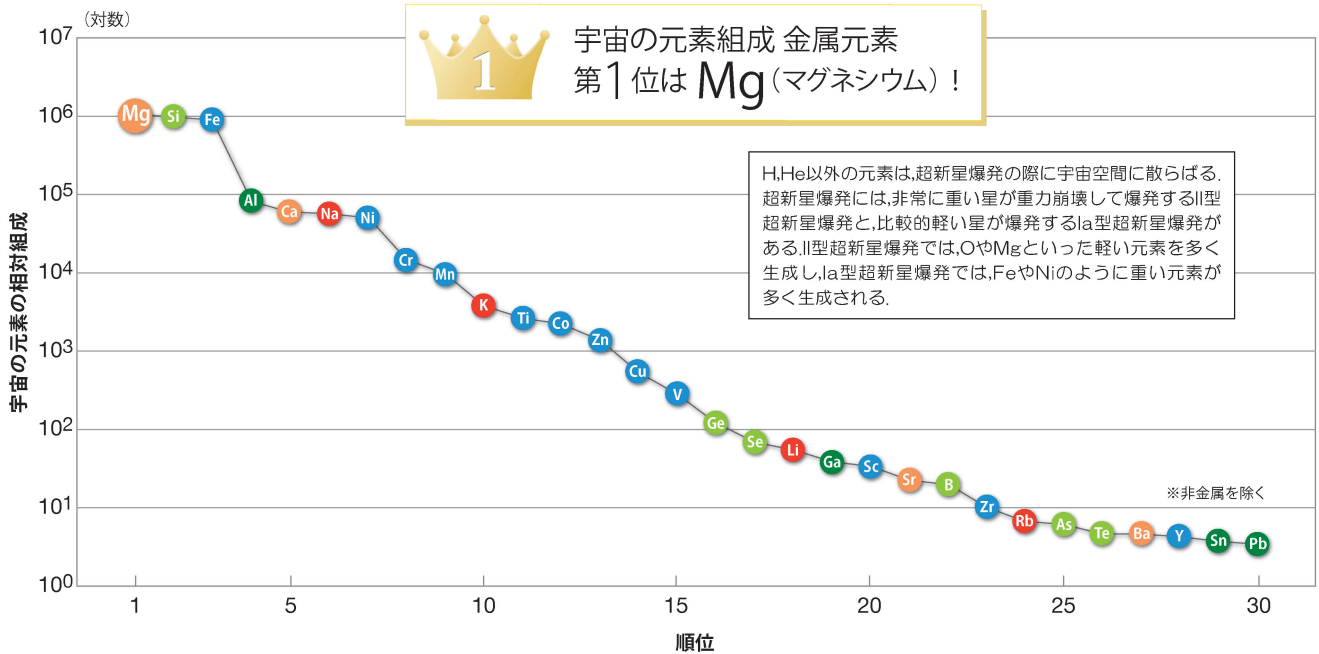
図2 宇宙の元素組成ランキング(30位まで).
