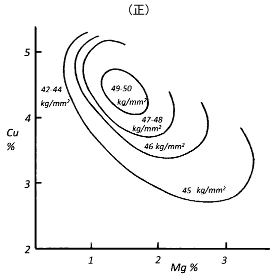
図1 ジュラルミン系合金の引張強さに及ぼす銅，マグネシウム添加量の影響 (20)(29)(30) 。
